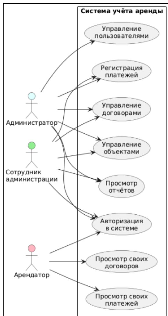
Рисунок 2 - UML-диаграмма
