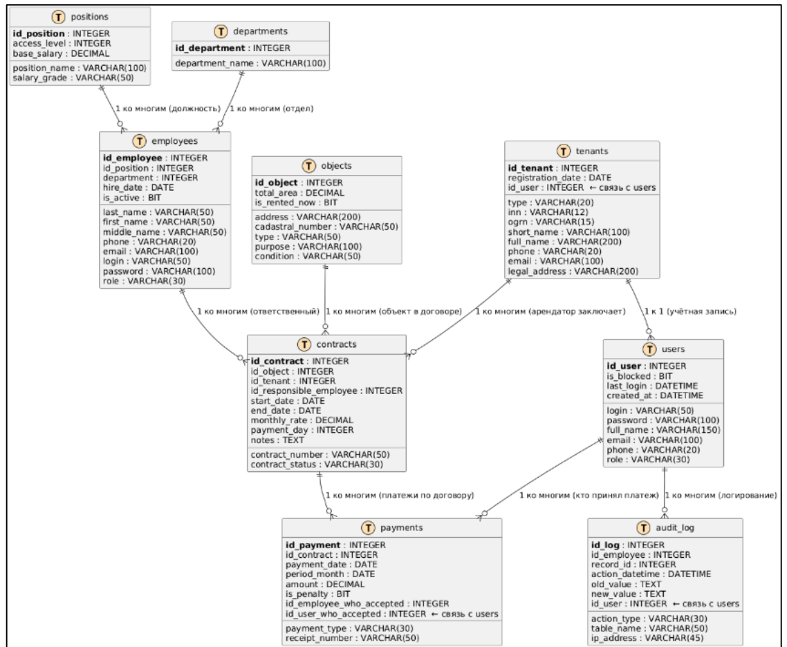
Рисунок 1 - ERD-диаграмма
