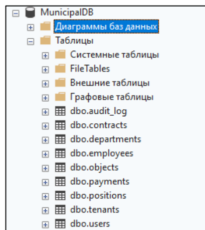
Рисунок 4 - Таблицы БД
