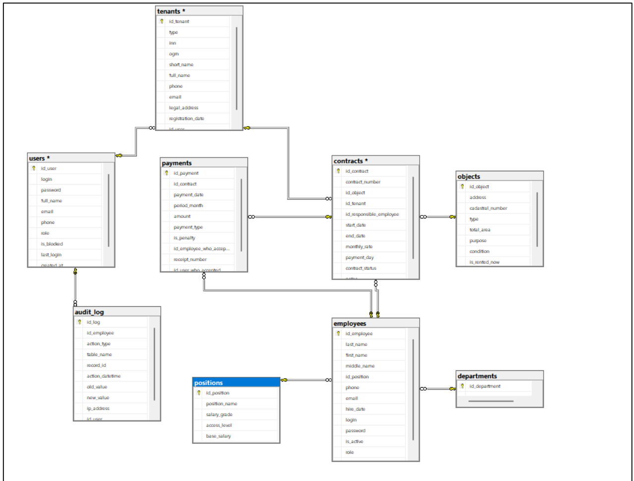
Рисунок 3 - Диаграмма БД
